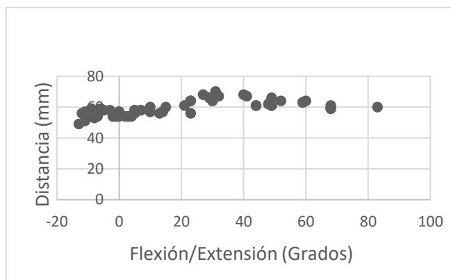
Fig. 5 –Brazo de palanca aplicado por el tendón rotuliano en rodilla sana.
