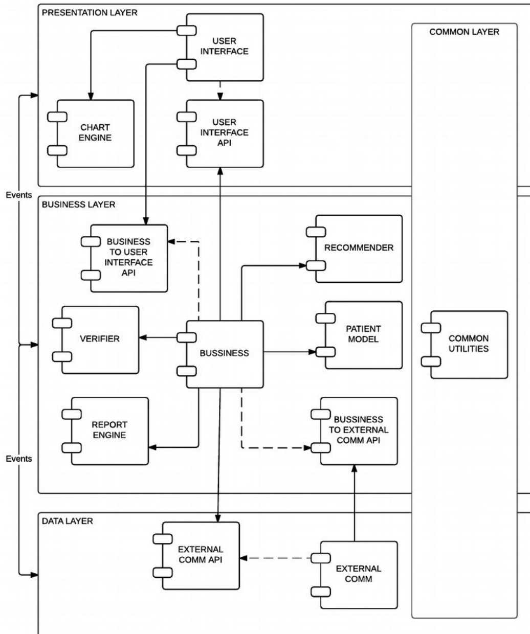
Figura 41 - Diagrama de arquitectura de SIMVENT-DOCEO.
