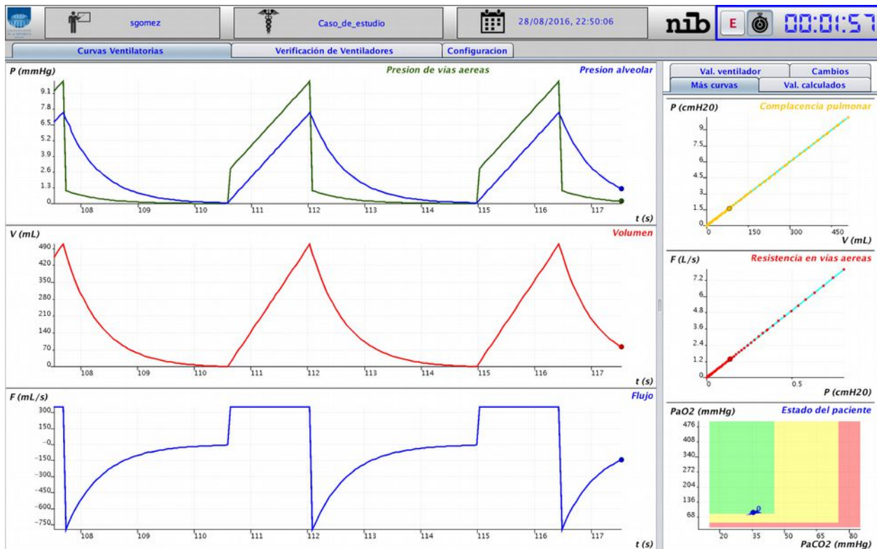
Figura 65 - SIMVENT-DOCEO con Simulador: Curvas ventilatorias y más curvas. Las curvas del simulador realizan una simulación casi perfecta en comparación con SIMVENT.
